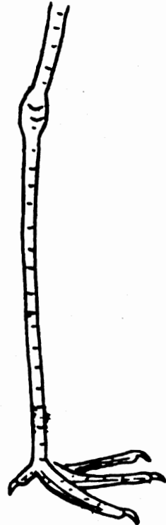
Wading Foot
